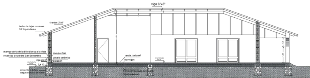
CASA C CORTE B-B
