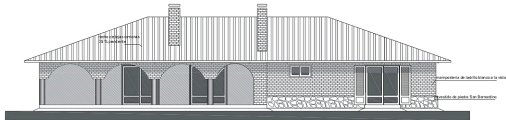
CASA C FACHADA POSTERIOR esc: 1/50
