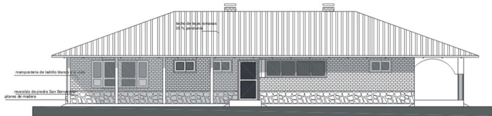
CASA C FACHADA PRINCIPAL esc: 1/50
