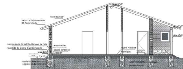
CASA C CORTE A-A
